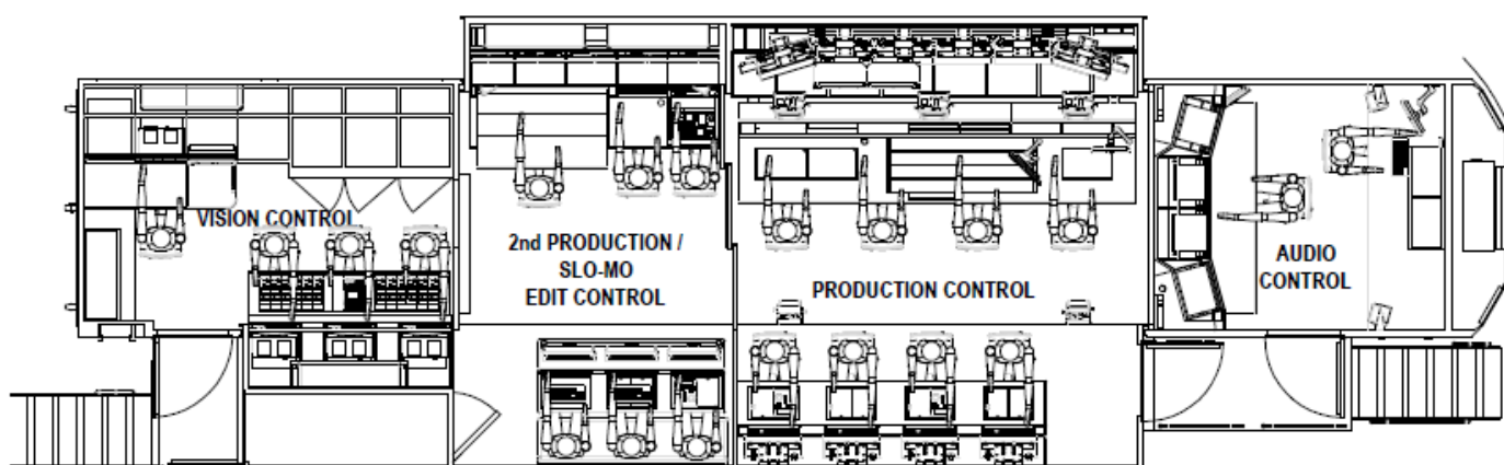
Layout reportažnega vozila HD-1
