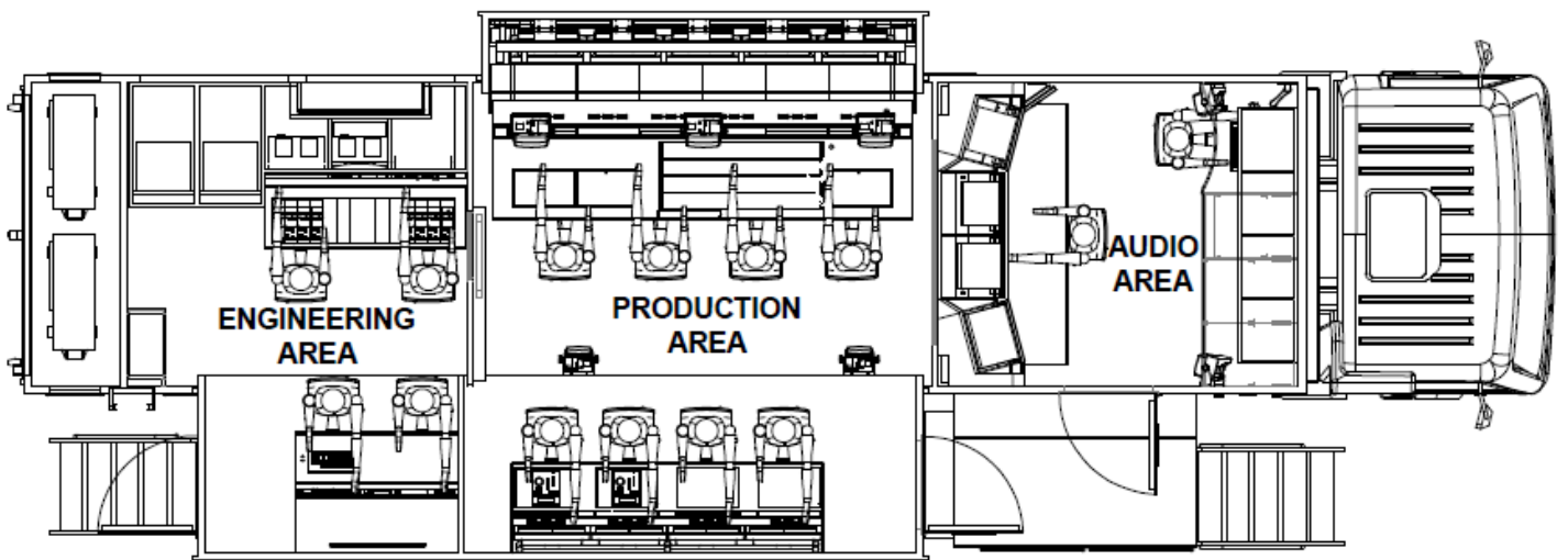
Layout reportažnega vozila HD-2
